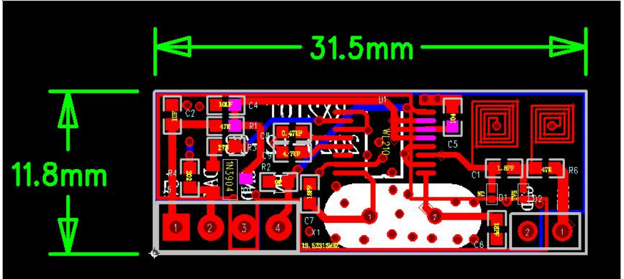
图 13 PCB 电路参考图
