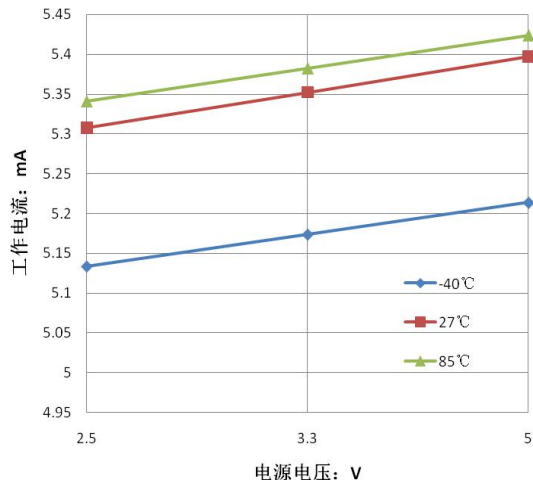
图9 . 433.92MHz时，三温电流随电压变化图
