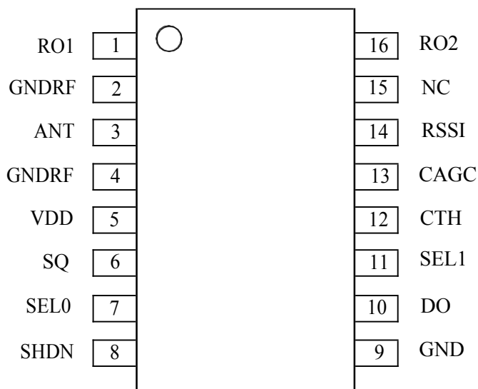
图2 WL219 SOP16L引出端排列
