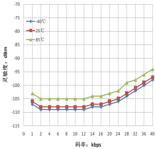
图7 433.92MHz时，三温灵敏度随码率变化图
