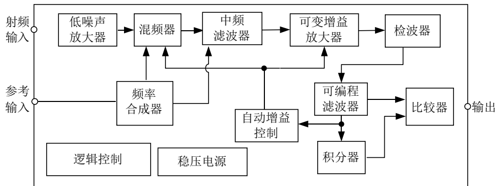
图 1 WL219 型 433MHz 短距离无线通讯接收机电路原理框图
